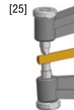
Chisel R 0,5 mm Plane Ø 3,5 mm
